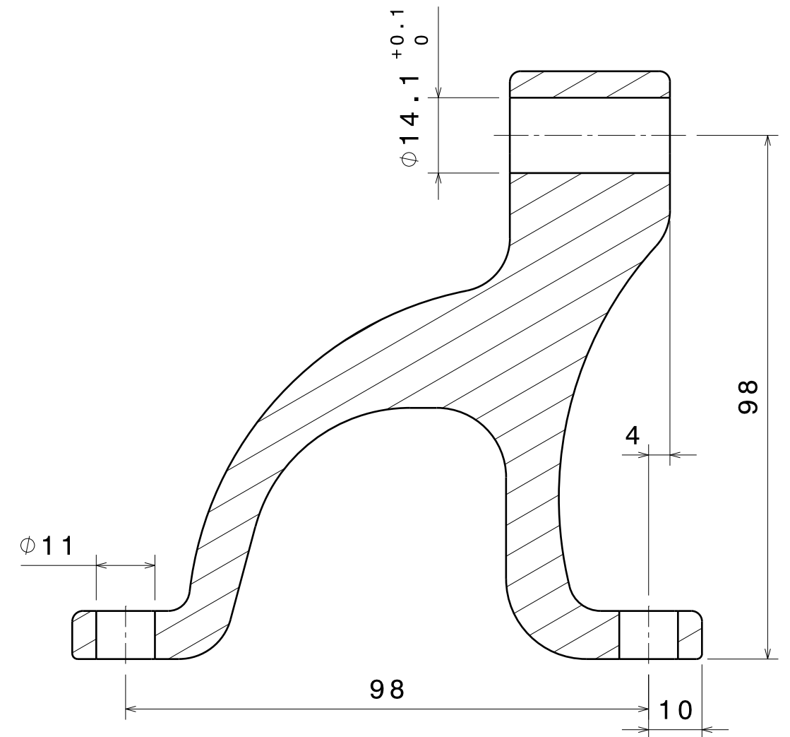
Schnitt A-A Maßstab: 1:1
